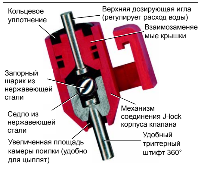
Рисунок 2В J-Lock
