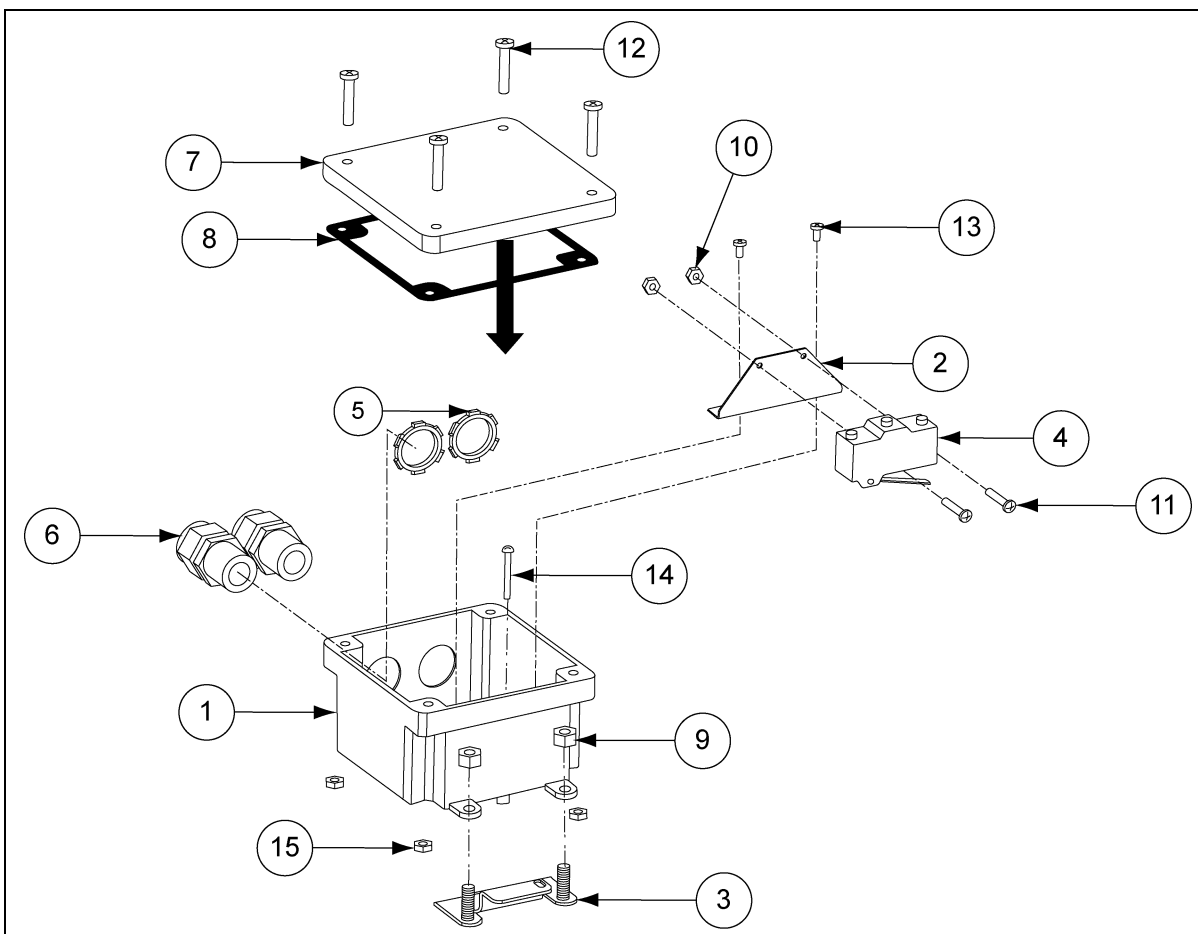
Электрошкаф концевого регулятора лотка в сборе, перечень деталей
