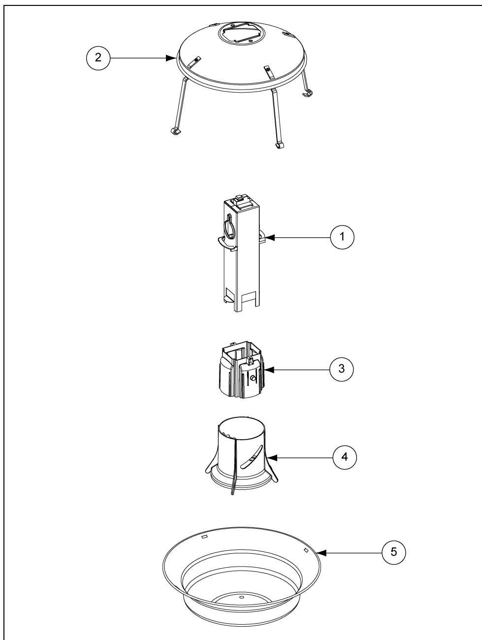
ATF Max в сборе, стальной лоток (C2000602), перечень деталей
