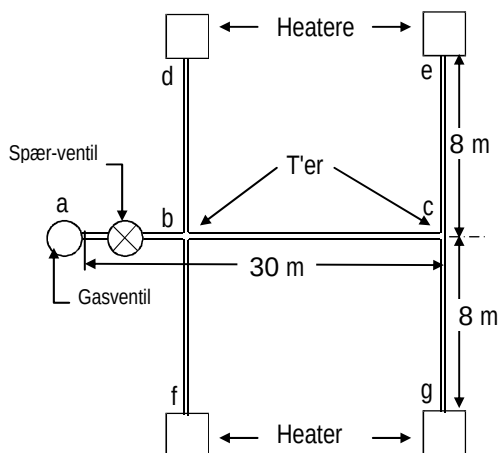
Eksempel på rørsystem
